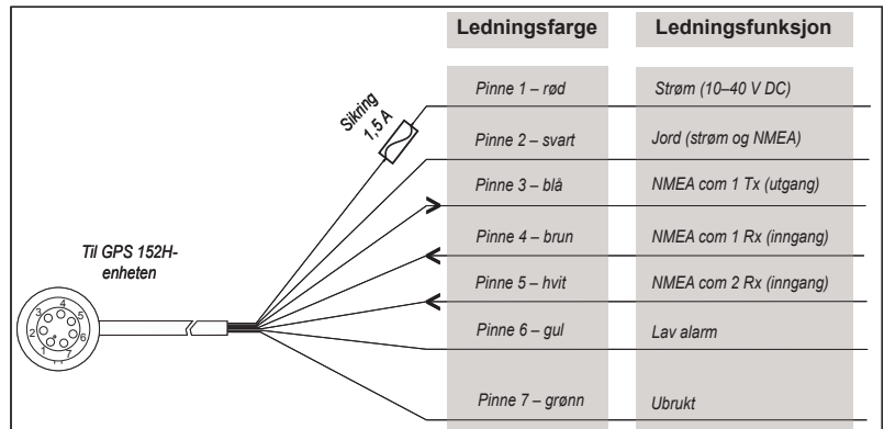
Ledningsnett for GPS 152H
